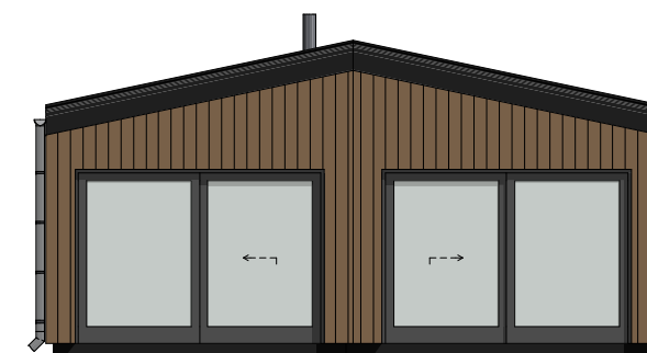
ELEWACJA FRONTOWA
