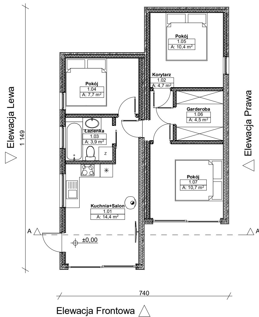
Elewacja Ogrodowa ▽
