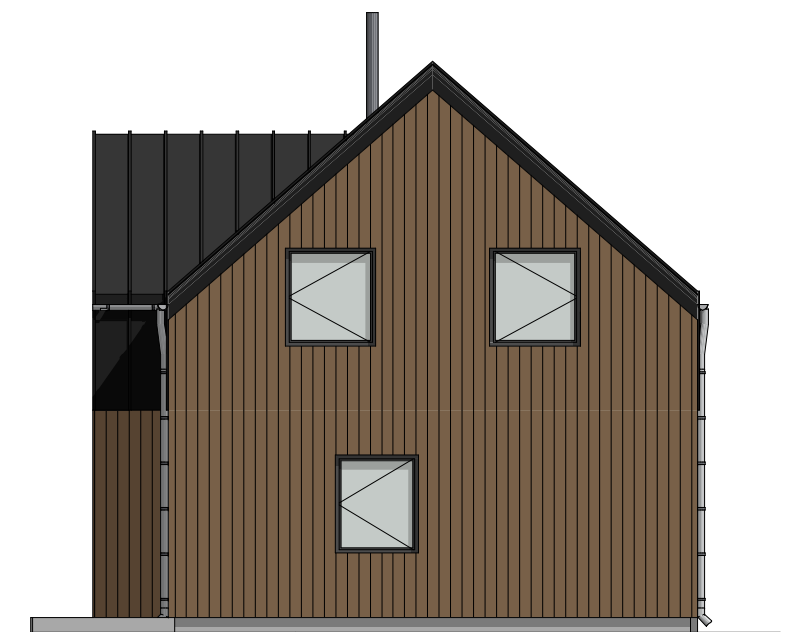
ELEWACJA PRAWA
