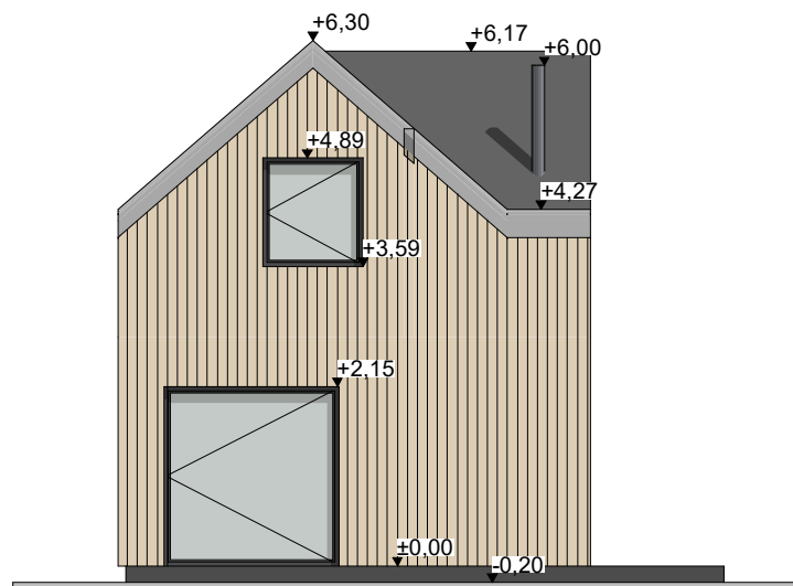
ELEWACJA LEWA
