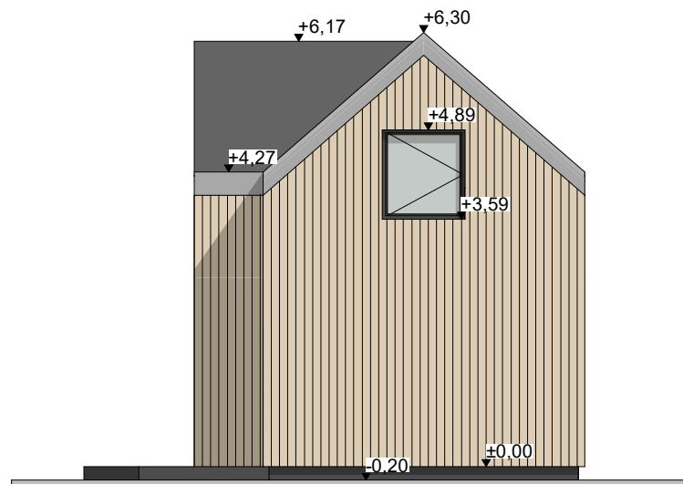
ELEWACJA PRAWA
