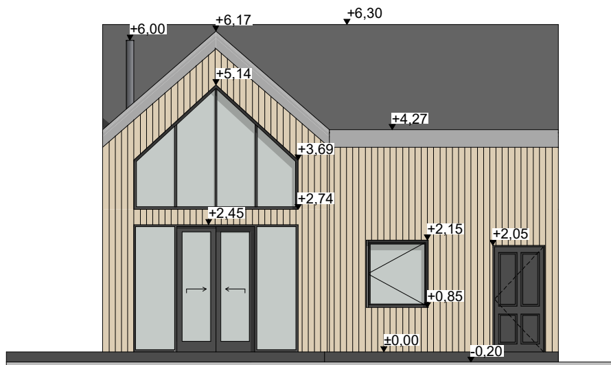
ELEWACJA FRONTOWA
