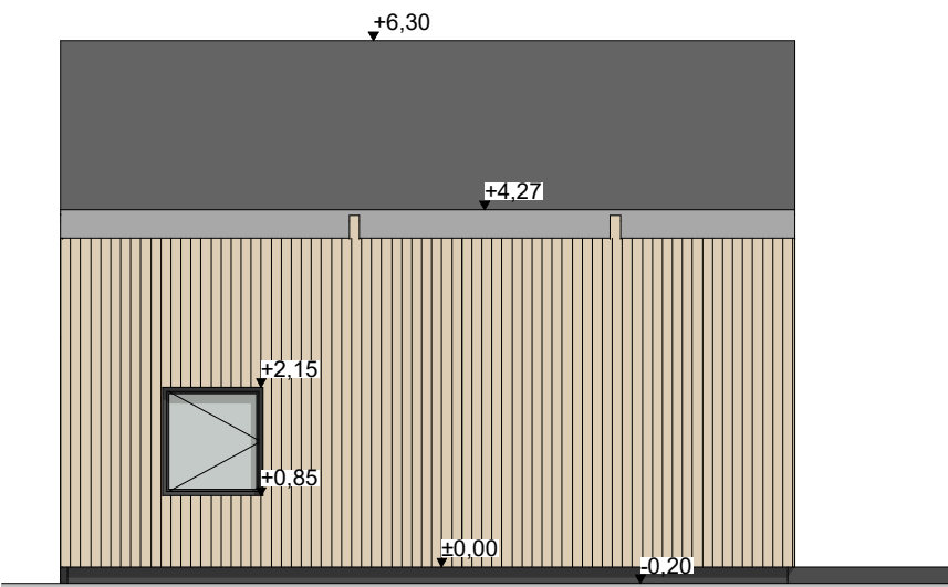
ELEWACJA TYLNA
